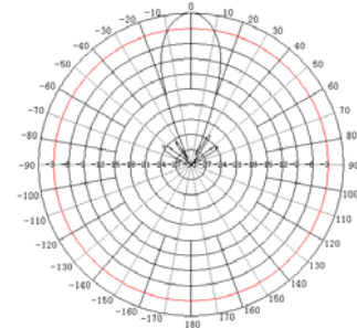
H-Plane
